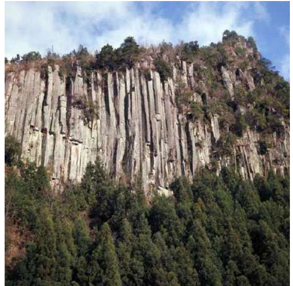
香落谷 花崗岩 柱状節理
